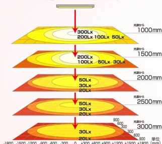
配光イメージ (1200T)
