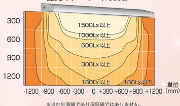
配光イメージ (1800L)
