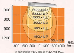
配光イメージ (600L)
