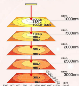
配光イメージ (600T)
